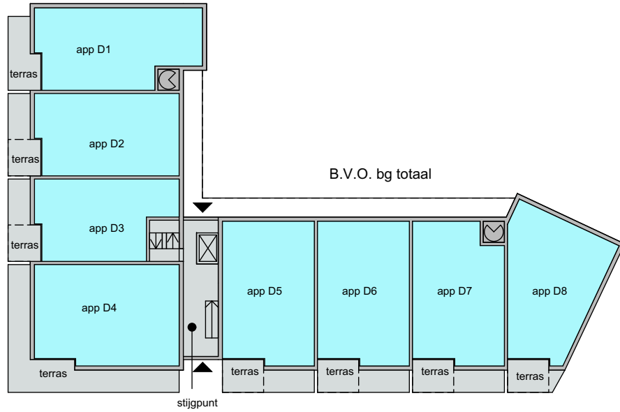
gebouw D b.g.
