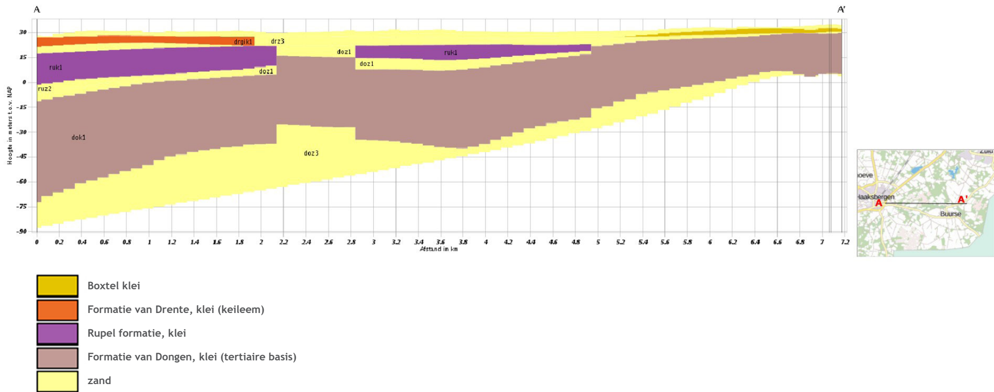
Figuur 3.2: dwarsdoorsnede van de weerstandslagen in de bodem op basis van diverse grondboringen. Keileem komt voor in het westelijke deel van het Buurserzand
