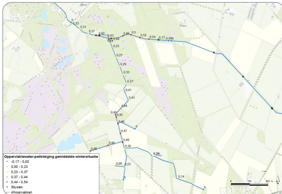
Figuur 4.3: Verwachte oppervlaktewaterpeilstijging in gemiddelde winter (vergunde situatie)
